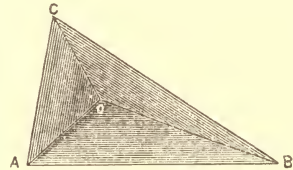
Fig. 4.—Trihedral Angle.
